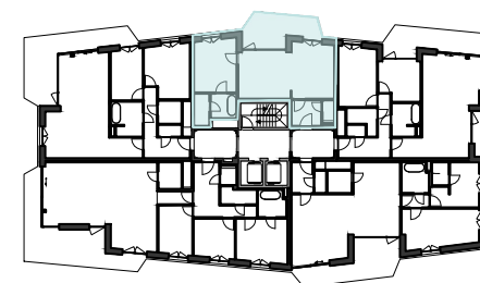
Verdiepingsplan +3
